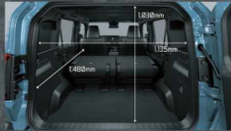
حيز الأمتعة
